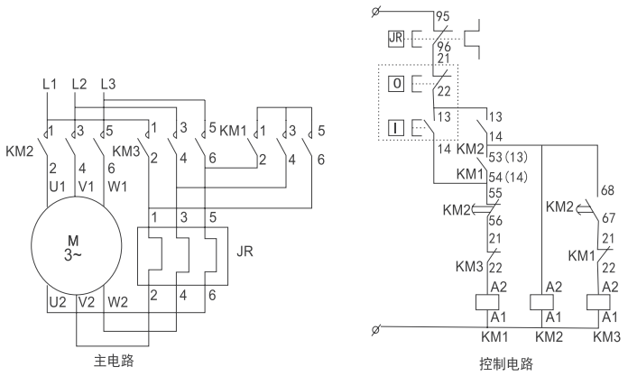
主电路和控制电路接线图
