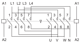
a. 控制可逆运转时接线图
