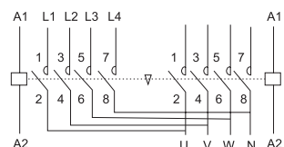
b. 控制双电源切换时接线图
