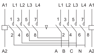
BC2N-1154~8004 配电用转换接触器
